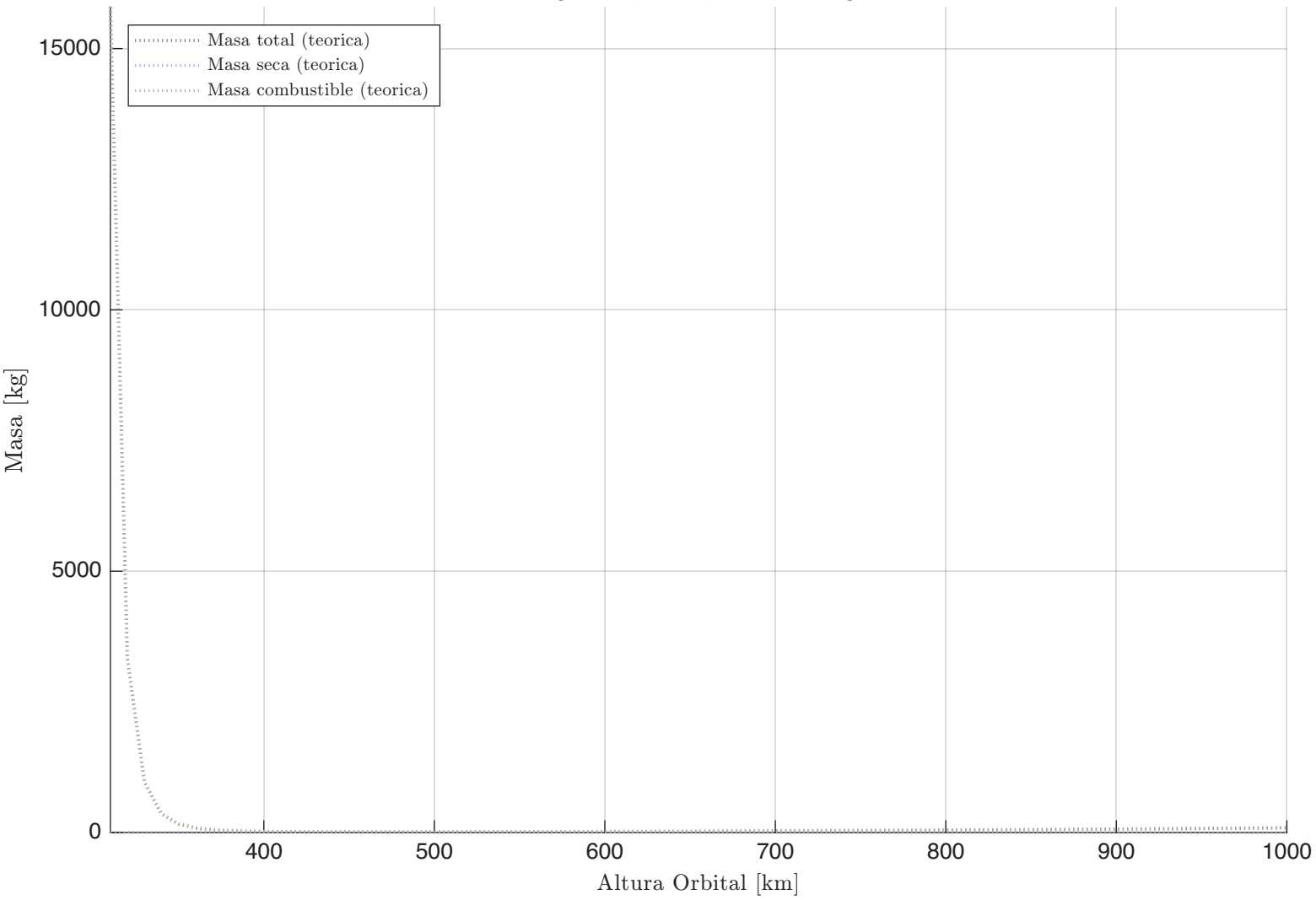
Desglose de Masas vs. Altura Config: 2 Sat, 2 Tel, Det 3, Cassegrain
